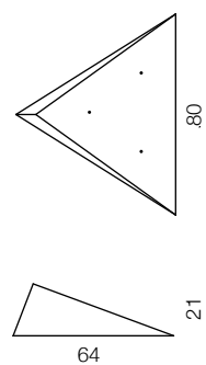
M 3 T-Nuts
