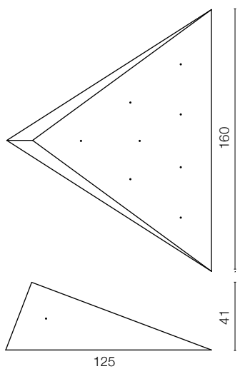
XL 10 T-Nuts
