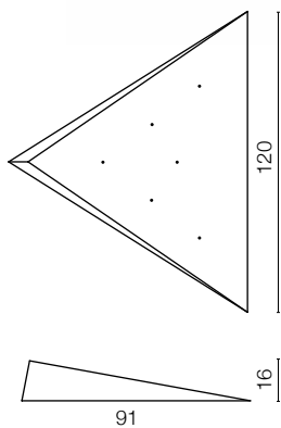
L 6 T-Nuts
